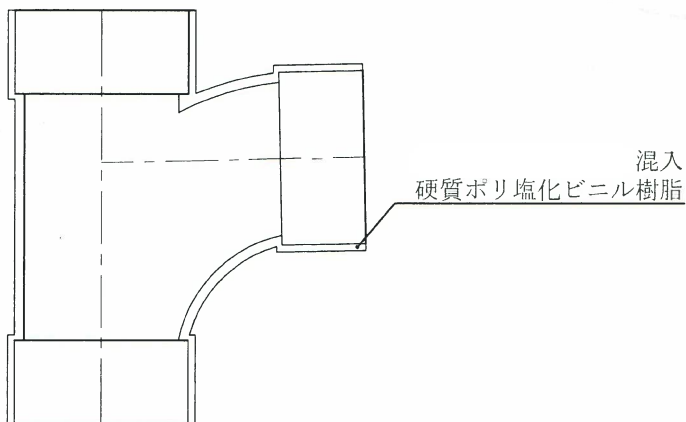
図-2 混入硬質ポリ塩化ビニル管継手の断面構造例
